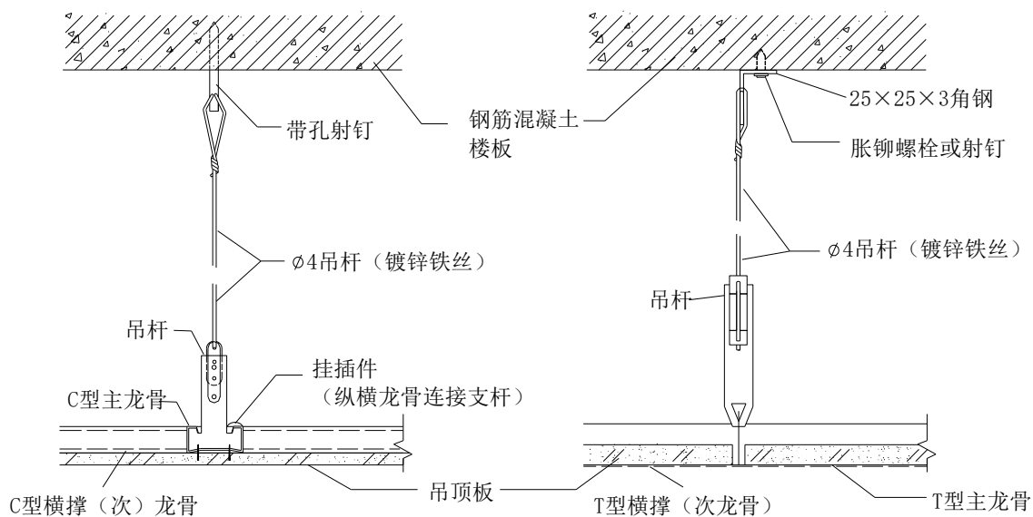
图 3.2.2.2(2) 不上人吊顶吊点紧固方式及悬吊构造节点
