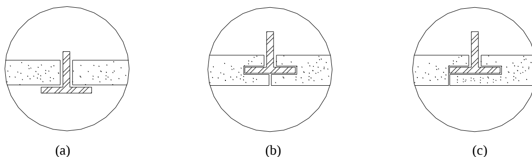
图 3.2.5.2 罩面板托卡固定法示意图
