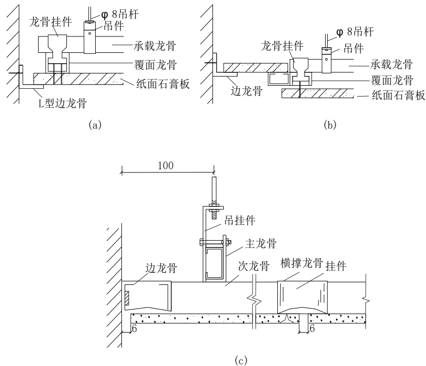
图 3.2.6 吊顶的边部节点构造
