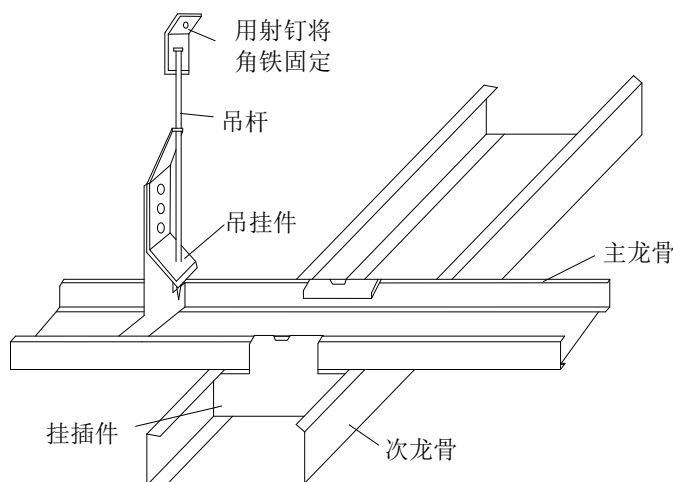
图 3.2.4 主、次龙骨连接
