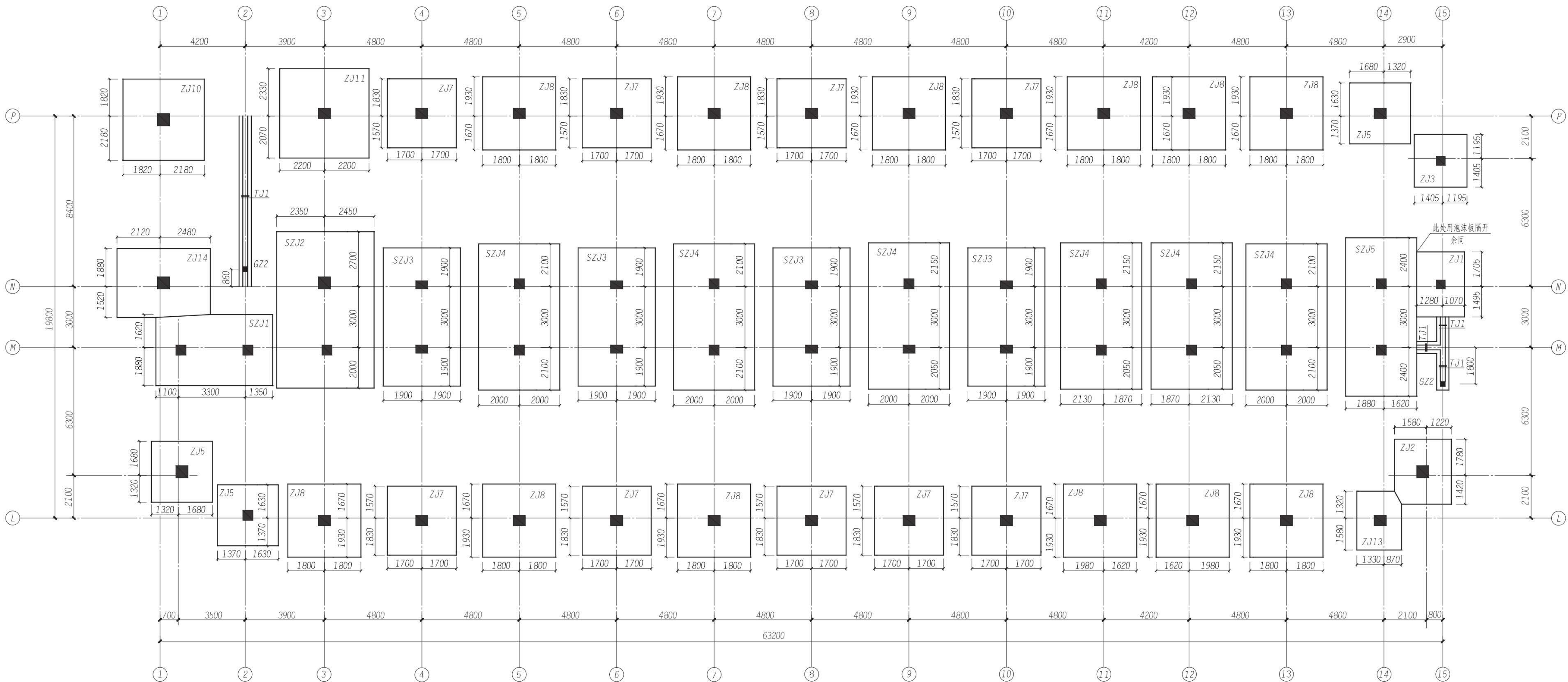
B区(L~P)轴基础平面布置图 1:100
