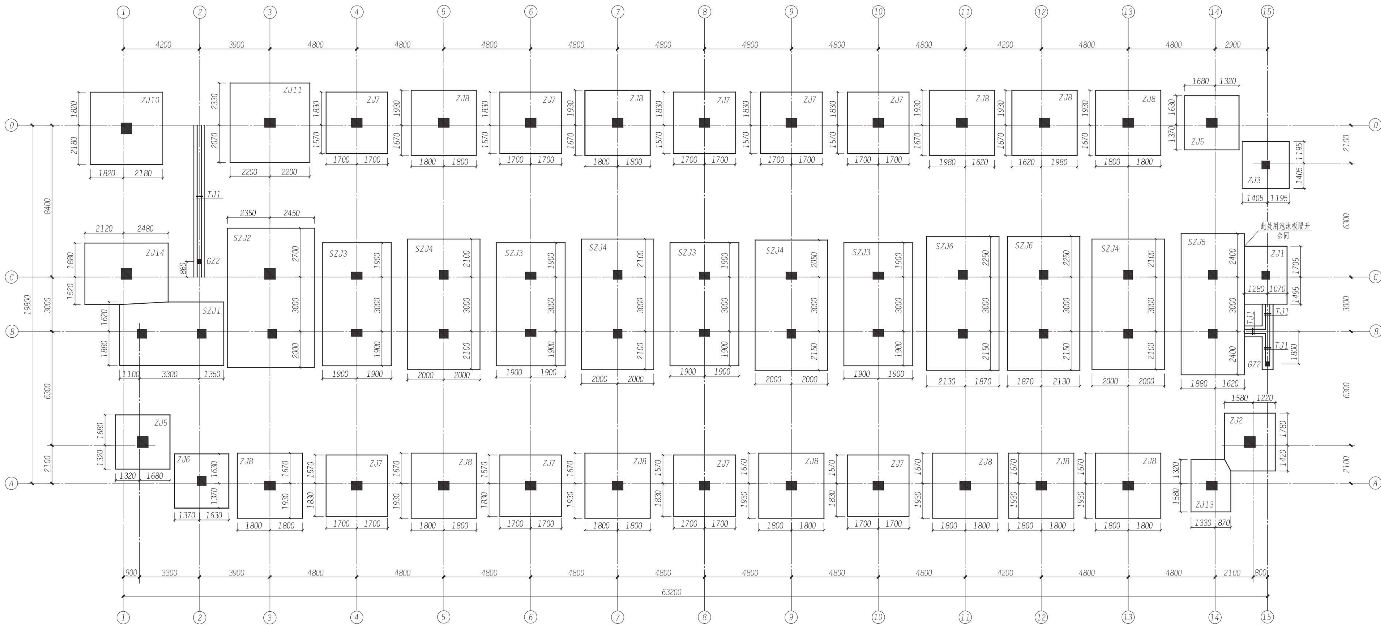
B区(A)~(D)轴基础平面布置图 1:100
