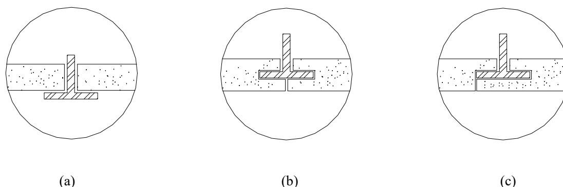
图 3.2.5.2 罩面板托卡固定法示意图
