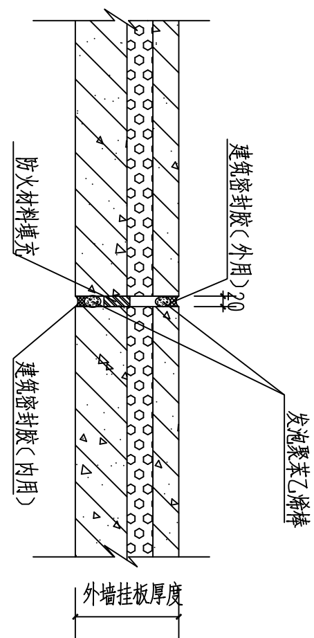
纵向缝
