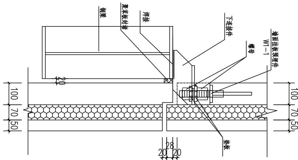
外墙挂板下部连接节点示意图
