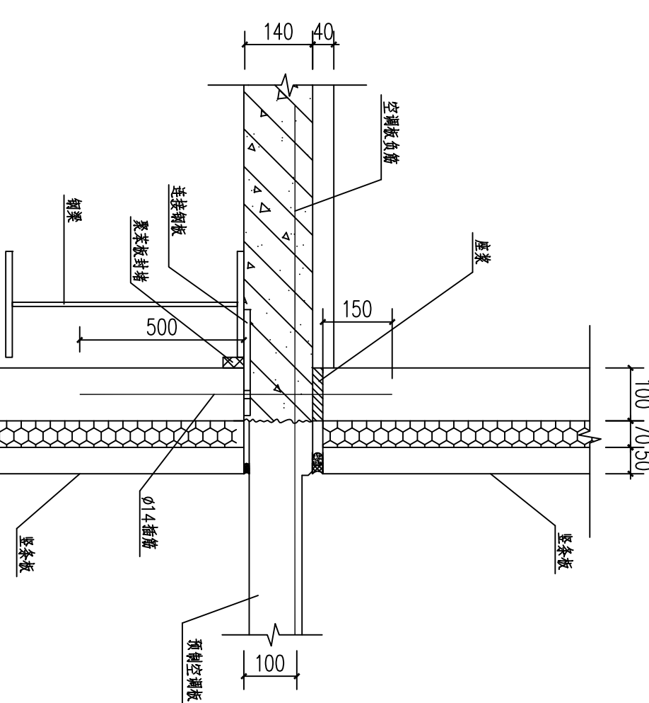
空调板板节点示意图
