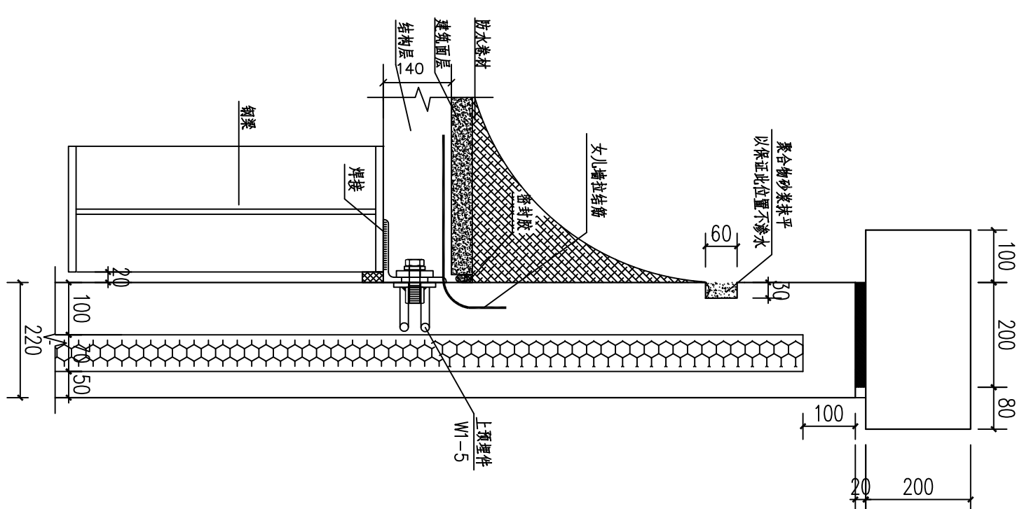
女儿墙与钢梁连接示意图
