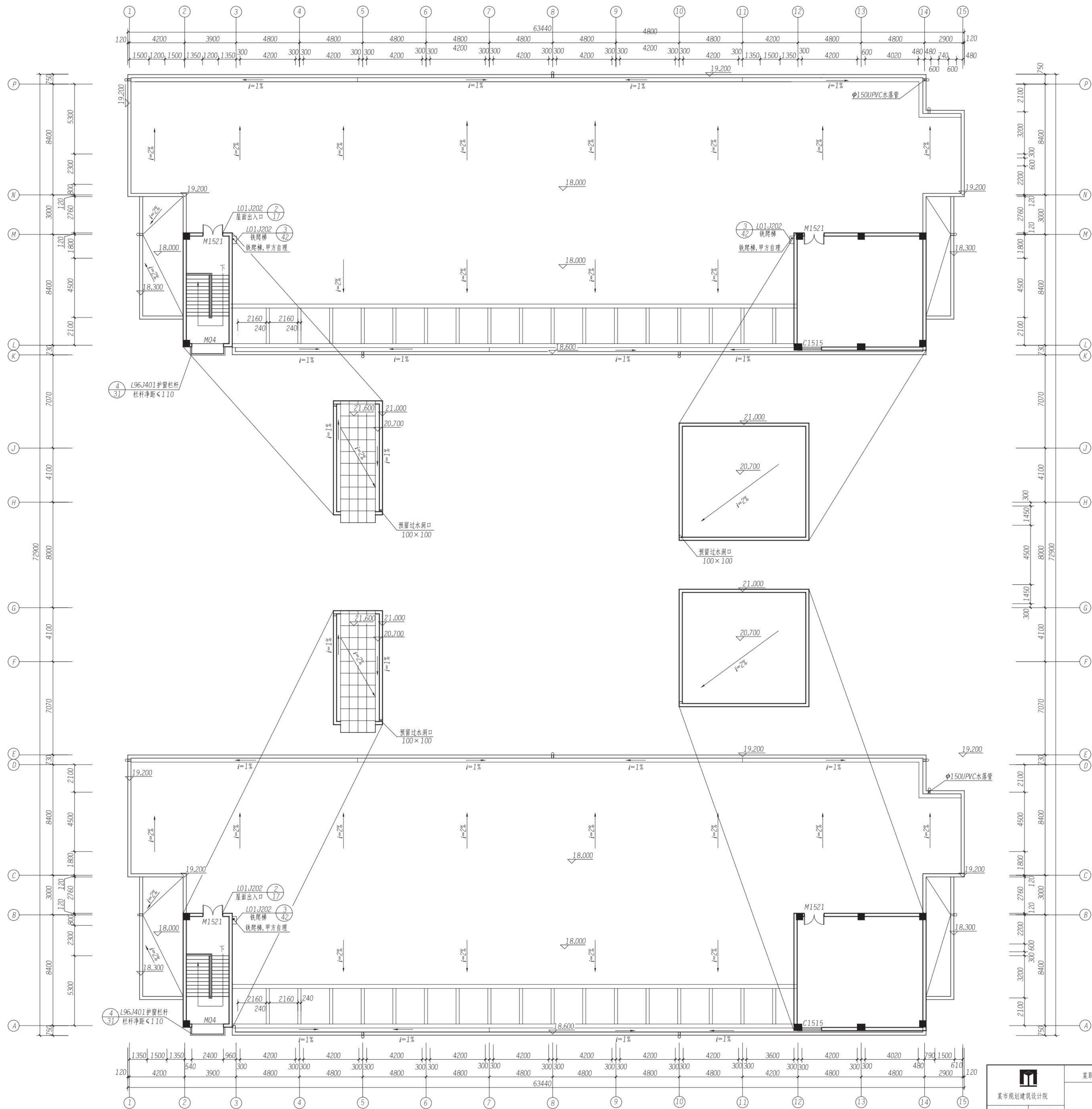
B区五层平面图 1:150
